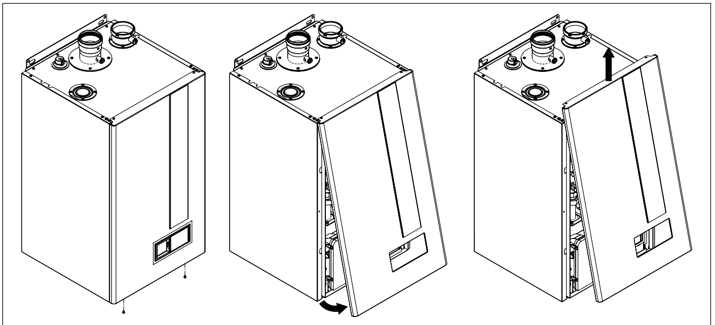
ábra 36 Burkolat nyitása
