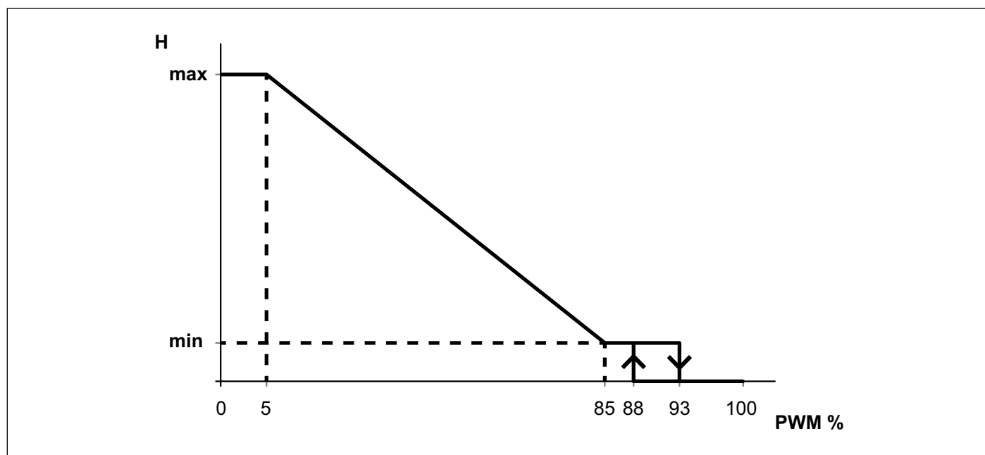
ábra 30 PWM jel
