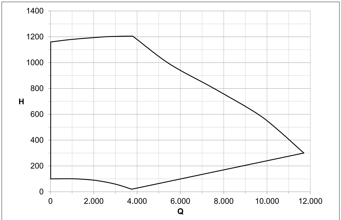
ábra 26 Rendelésre álló emelőmagasság YONOS PARA HF 25/12
