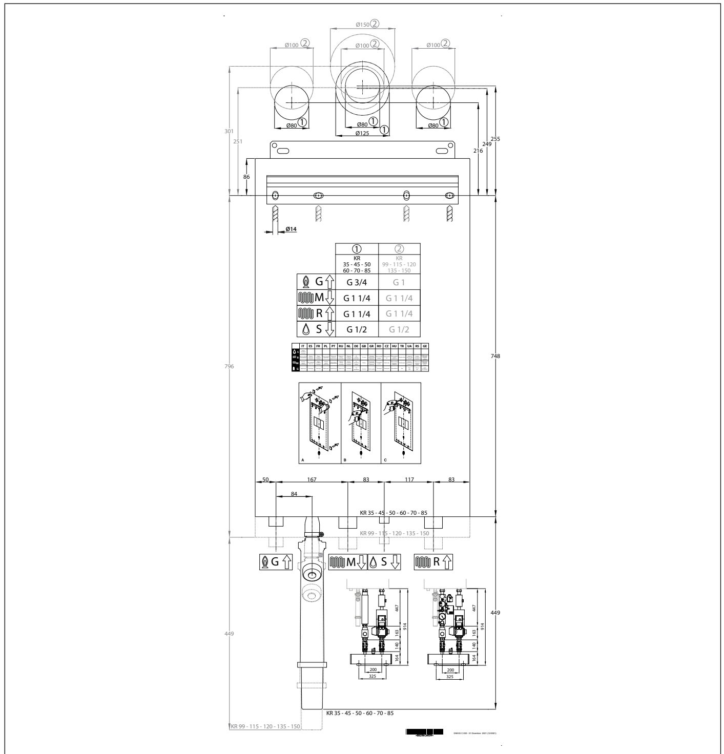
ábra 10 Rögzítősablon
