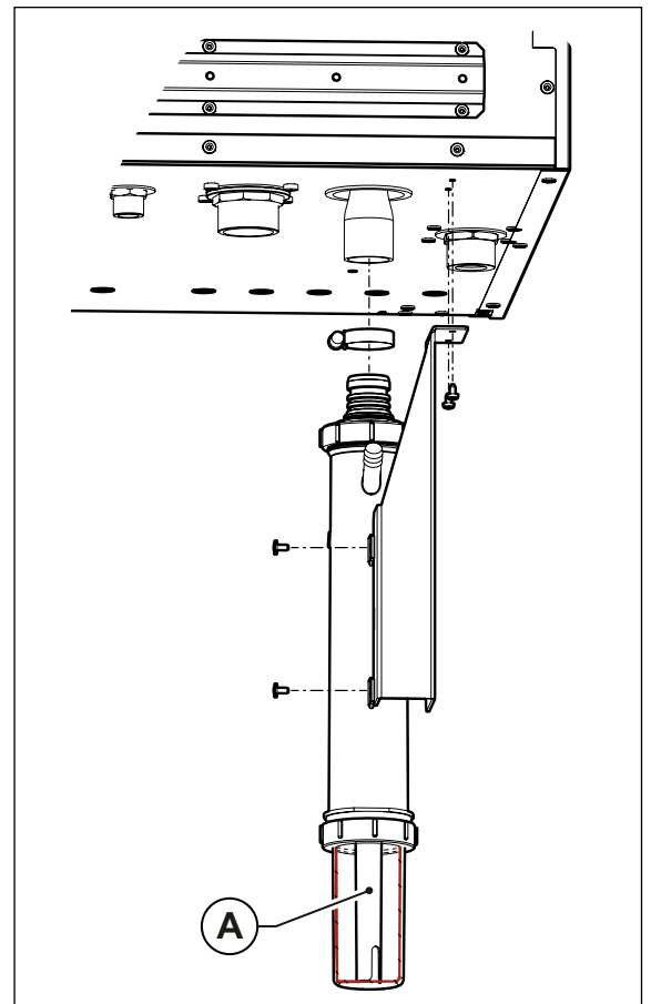
ábra 11 A csapda rögzítése
