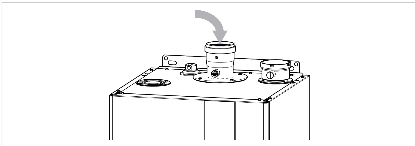
ábra 42 Szifon feltöltése
