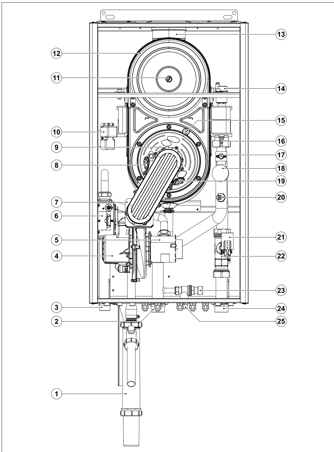
ábra 7 Részegységek KR 120 (I)
