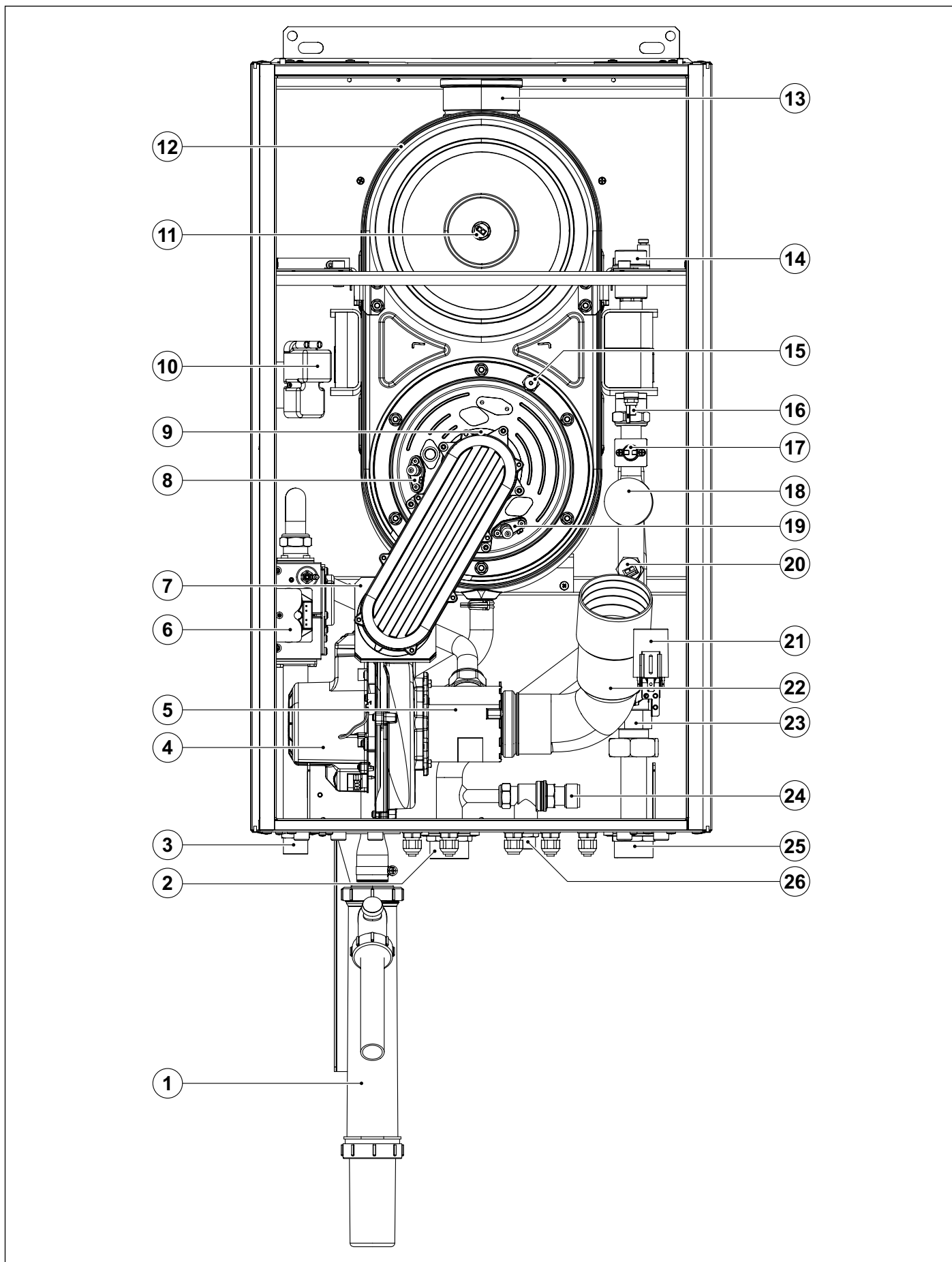
ábra 5 Részegységek KR 85 (I)
