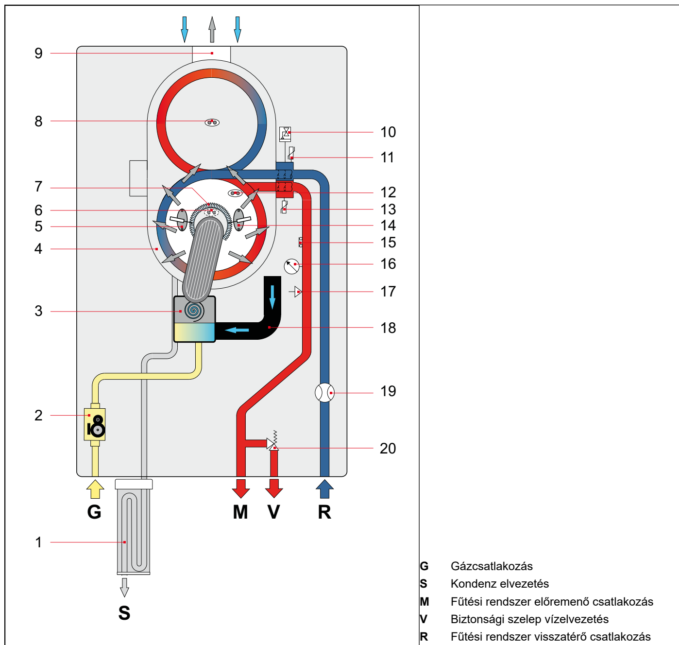
ábra 9 Hidraulikai vázlat
