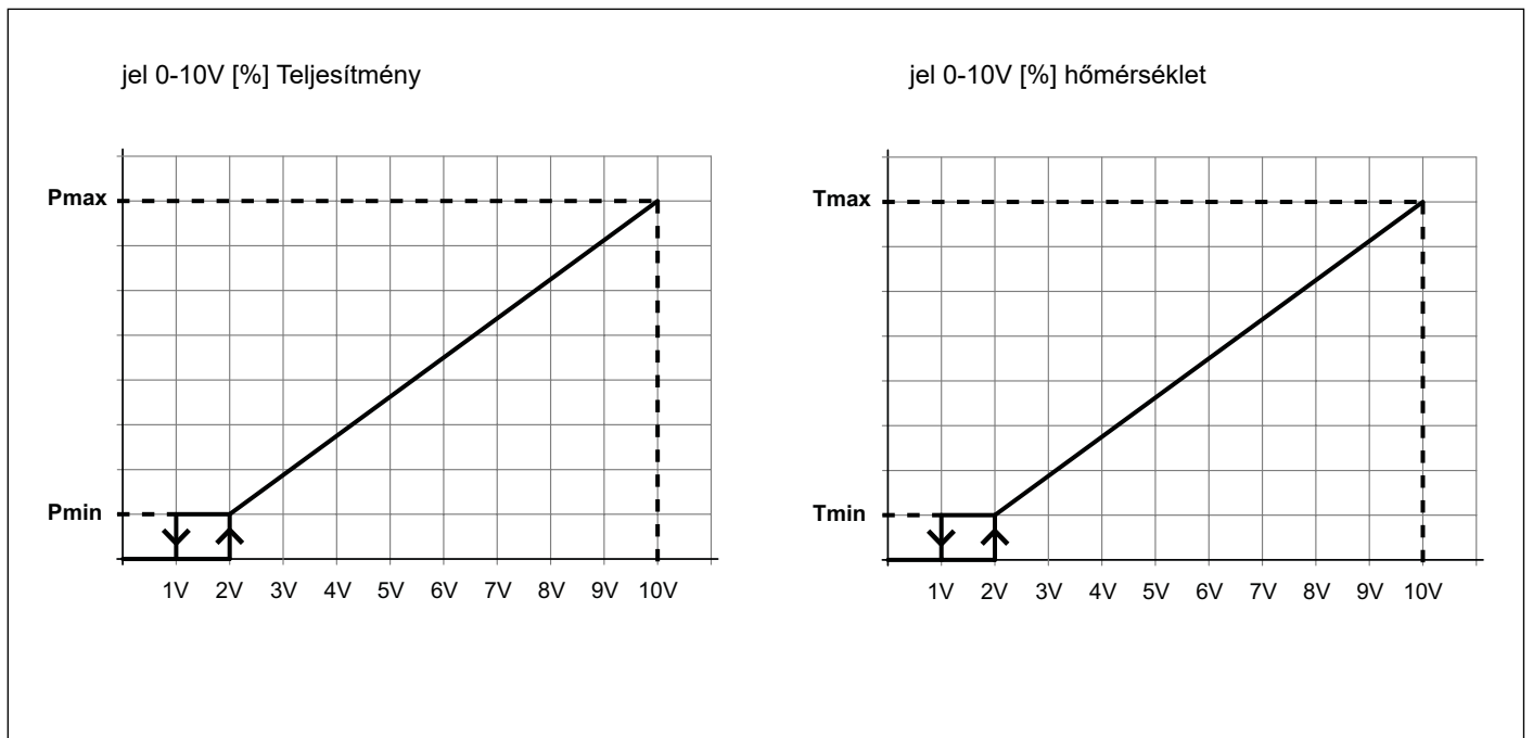
ábra 21 jel 0-10 VDC
