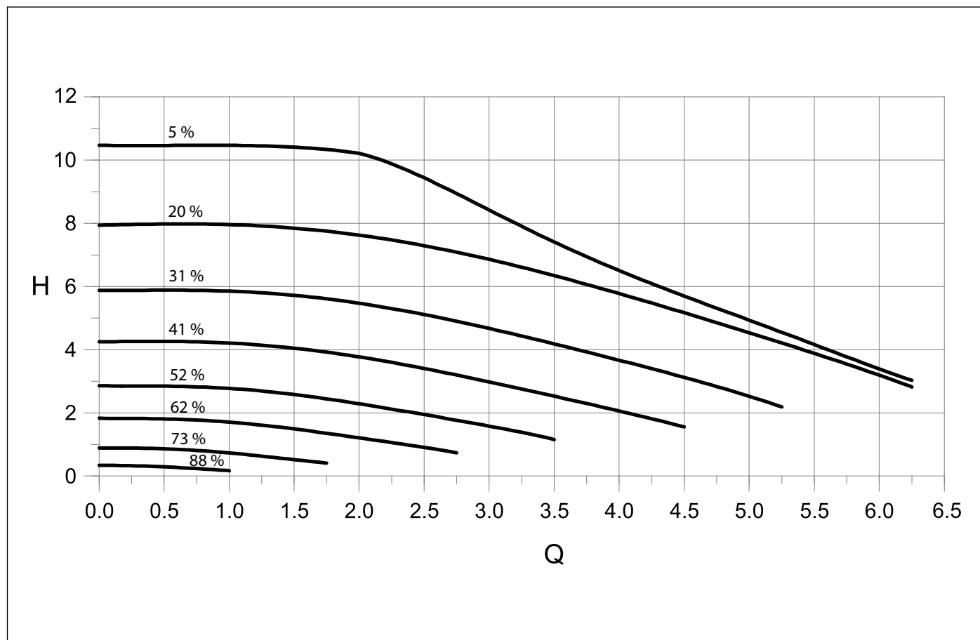
ábra 27 Rendelésre álló emelőmagasság UPML 25 - 105 - 180 PWM
