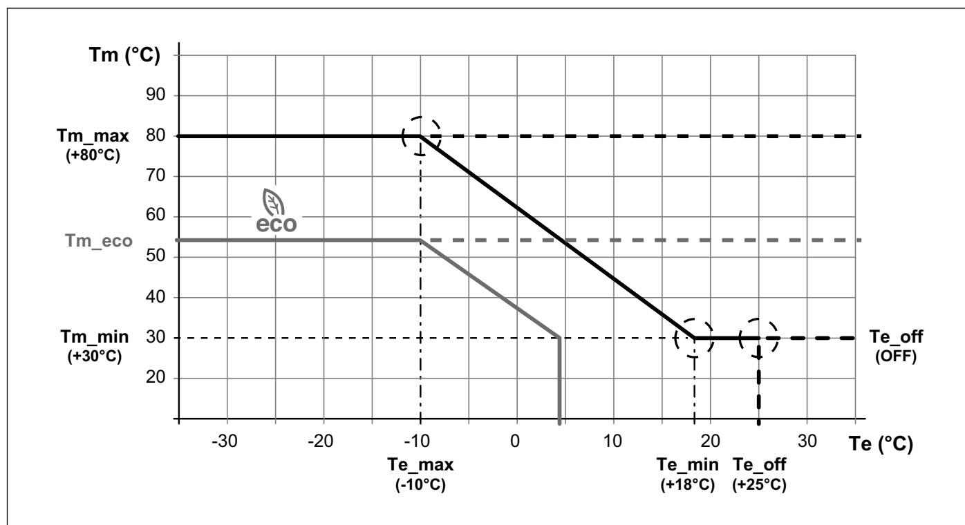
ábra 20 Időjárásfüggő jelleggörbe
