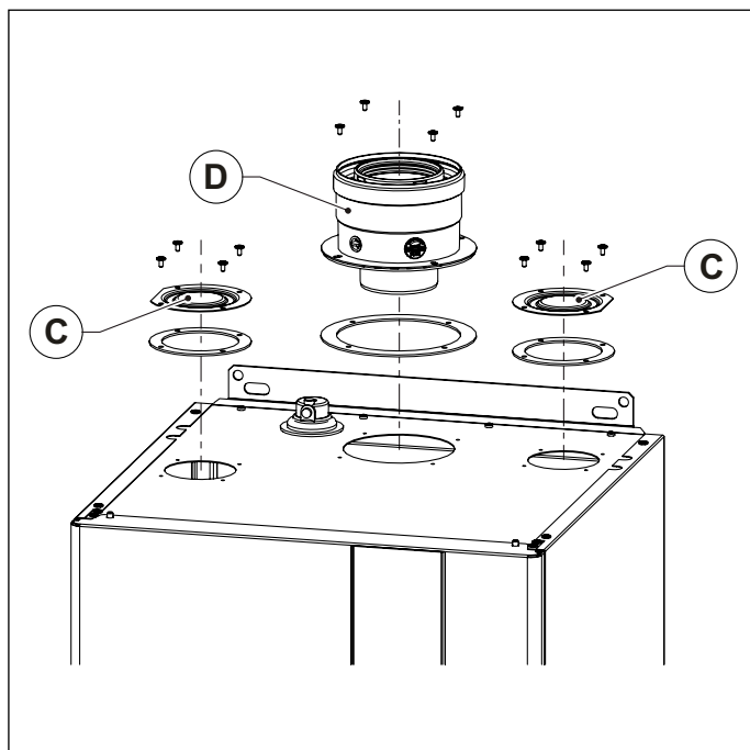
ábra 13 Koncentrikus indítódóm
