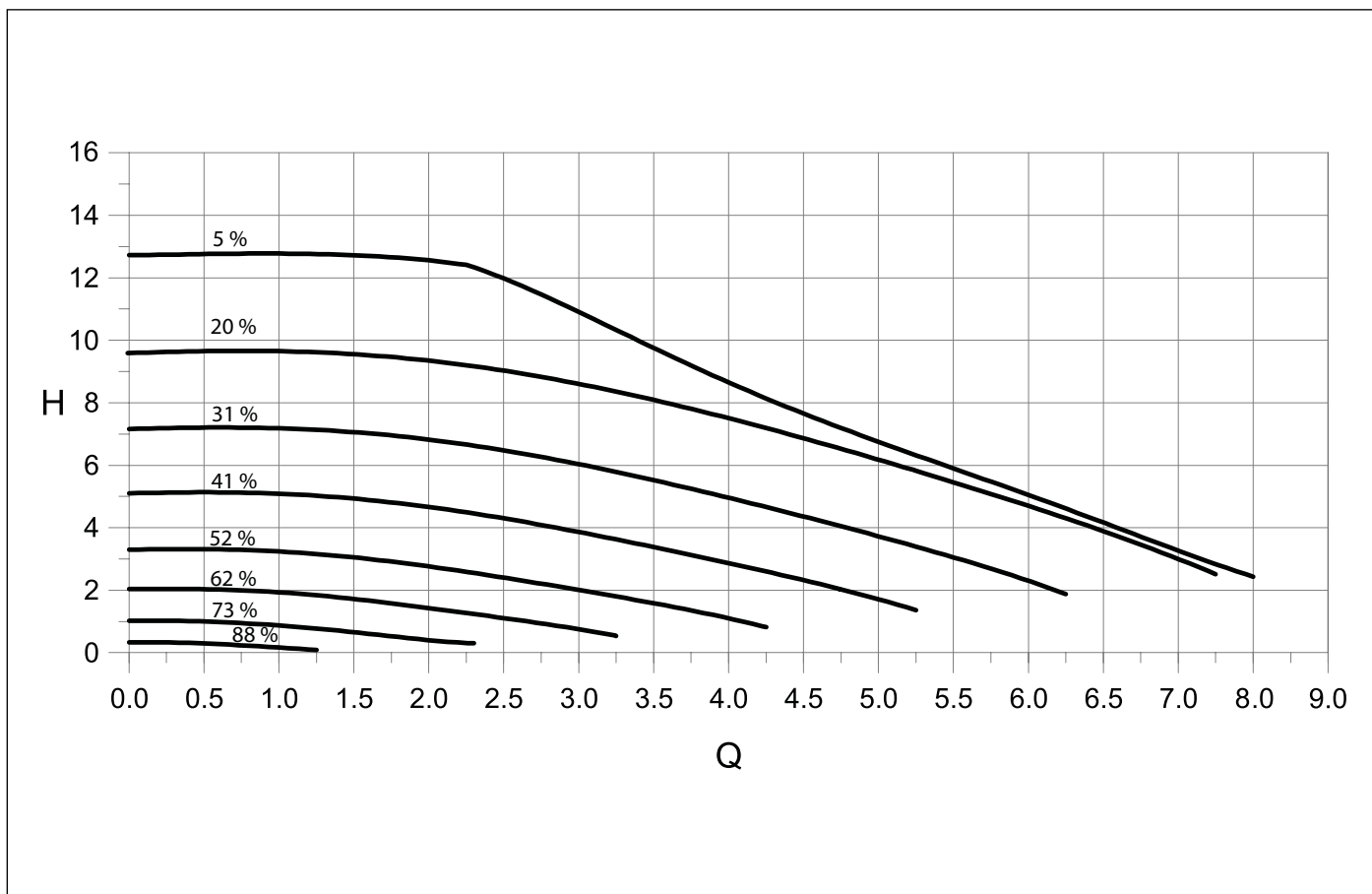
ábra 28 Rendelésre álló emelőmagasság UPMXL 25 - 125 - 180 PWM
