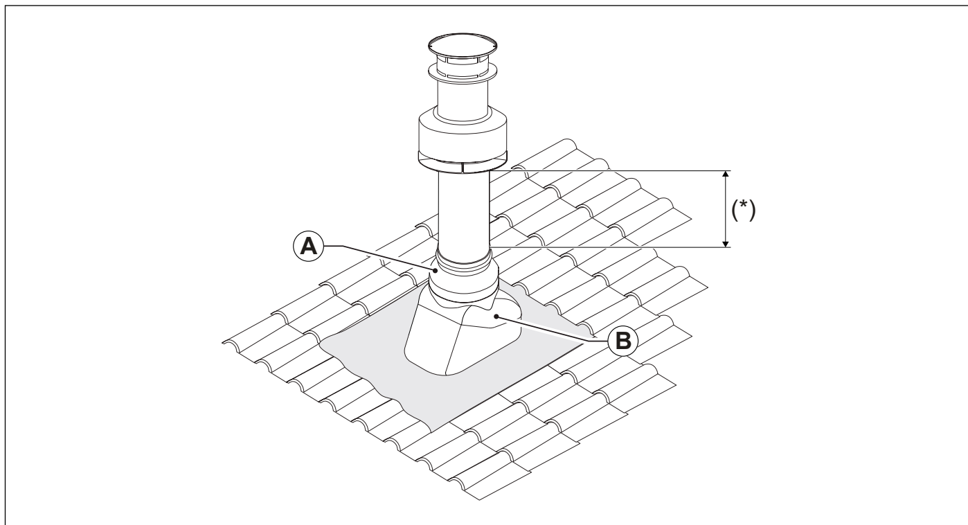
ábra 18 A függőleges végelem telepítése
