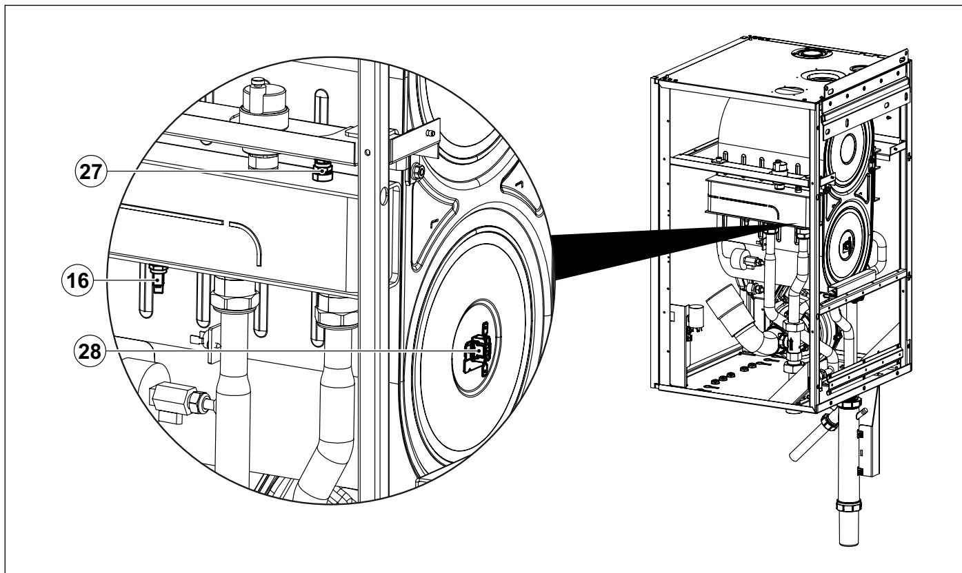
ábra 6 Részegységek KR 85 (II)
