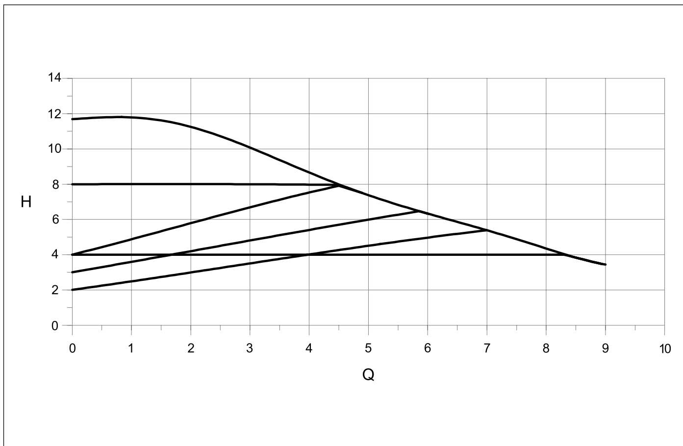
ábra 29 Rendelésre álló emelőmagasság UPMXXL 25 - 120 - 180 AUTO
